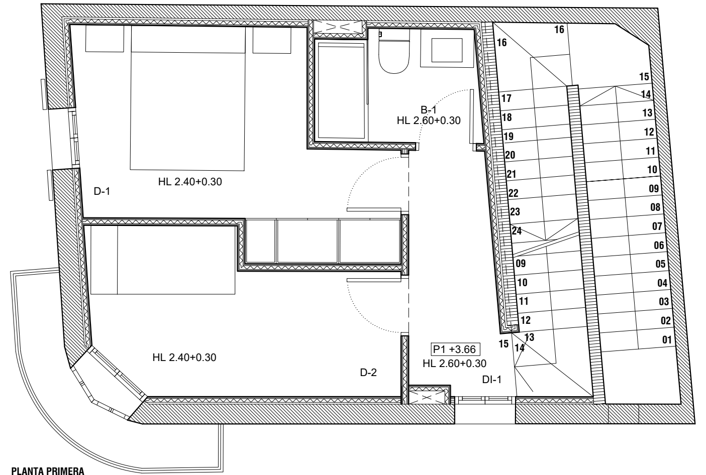
PLANTA PRIMERA
