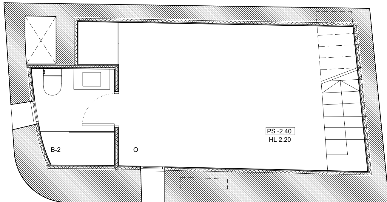
PLANTA SÓTANO
